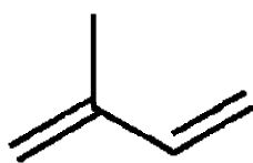
isoprene
